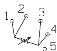
四线热电阻以及欧姆
