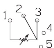
3 线制热电阻和欧姆 (1)
