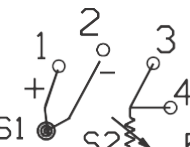
\Delta T /热备份/带热电阻/热电偶的双传感器 (1)
