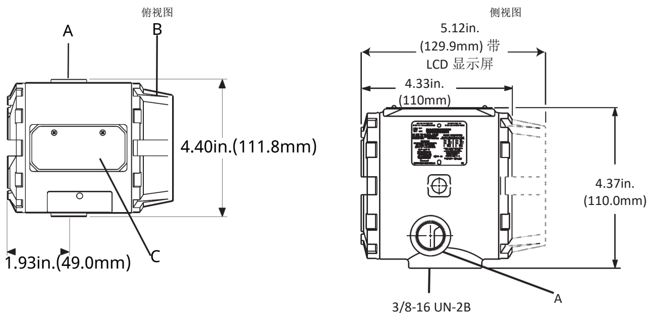
图 4: 变送器视图
