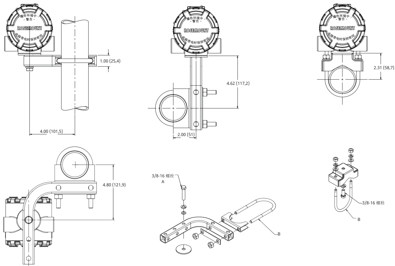
图 6：使用可选安装架的管道安装配置
