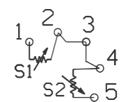
\Delta T /热备份/带两个热电阻和补偿回路的双传感器 (1)
